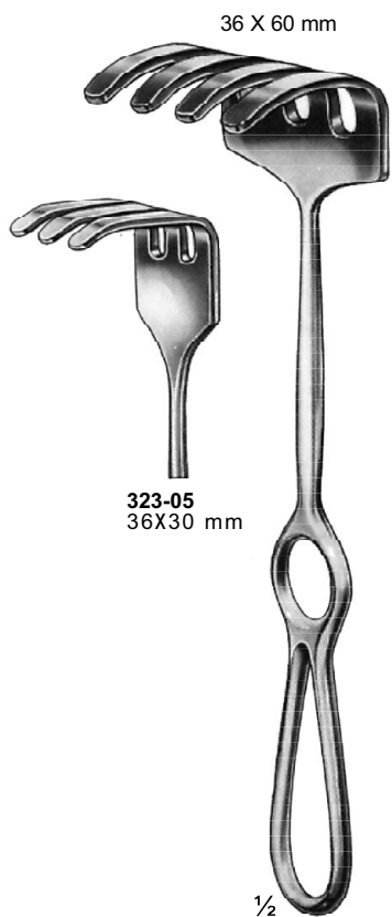
Ollier 323-05 36X30 mm 323-06 36X60 mm 23 cm / 9"
