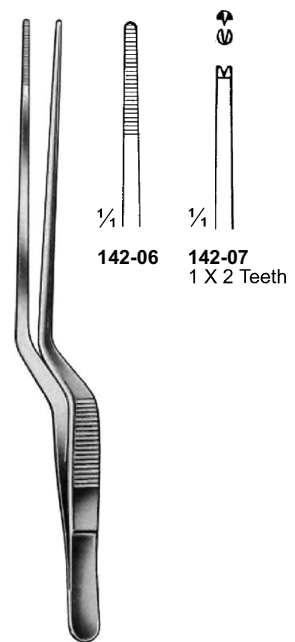
Gruenwald (Jansen) 142-06 & 142-07 16 cm / 6¼"
